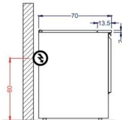
Vista Izquierda
