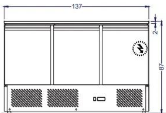
Vista Elevación
